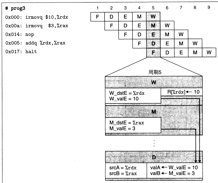
图 4-50 prog3 使用转发的流水线化的执行。在周期 5 中，译码阶段逻辑发现有在写回阶段中对寄存器 %rdx 未进行的写，以及在访存阶段中对寄存器 %rax 未进行的写。它用这些值，而不是从寄存器文件中读出的值，作为 valA 和 valB 的值
