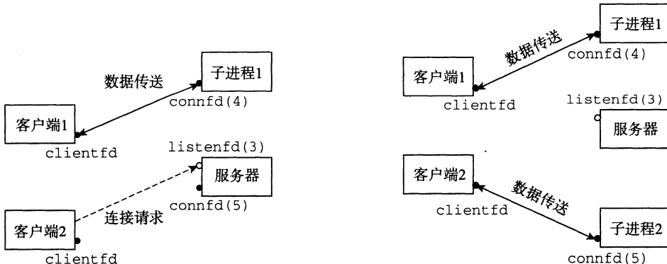
图 12-3 第三步：服务器接受另一个连接请求 图 12-4 第四步：服务器派生另一个子进程为新的客户端服务
