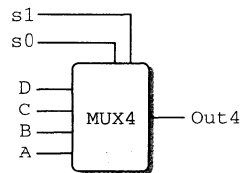
图 4-14 四路复用器。控制信号 s1 和 s0 的不同组合决定了哪个数据输入会被传送到输出
