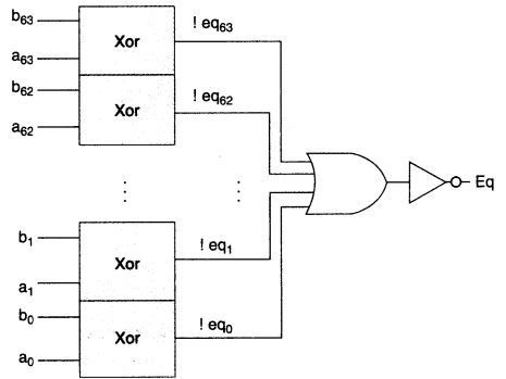
图 4-71 练习题 4.10 的答案
