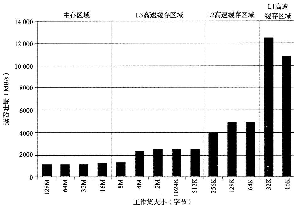
图 6-42 存储器山中时间局部性的山脊。这幅图展示了图 6-41 中 stride=8 时的一个片段
