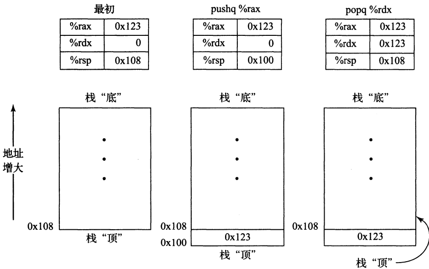
图 3-9 栈操作说明。根据惯例，我们的栈是倒过来画的，因而栈“顶”在底部。x86-64 中，栈向低地址方向增长，所以压栈是减小栈指针（寄存器 %rsp ）的值，并将数据存放到内存中，而出栈是从内存中读数据，并增加栈指针的值
