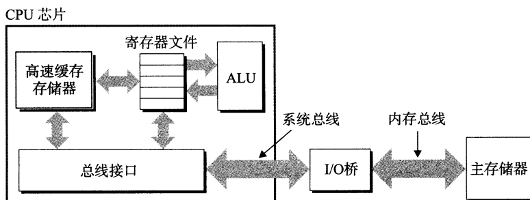
图 1-8 高速缓存存储器
