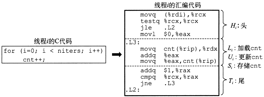
图 12-17 badcnt.c 中计数器循环(第 40~41 行)的汇编代码
