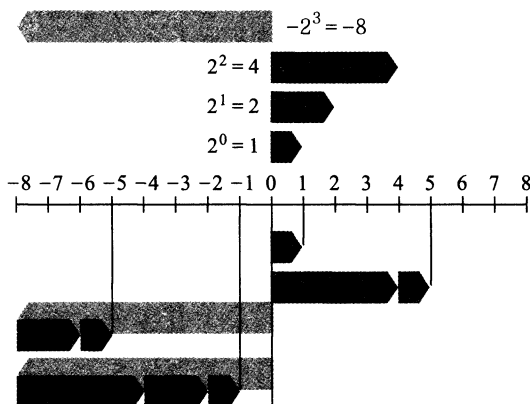
图 2-13 w=4 的补码示例。把位 3 作为符号位，因此当它为 1 时，对数值的影响是 -2^3 = -8 。这个权重在图中用带向左箭头的条表示
