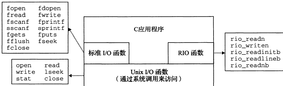
图 10-16 Unix I/O、标准 I/O 和 RIO 之间的关系
