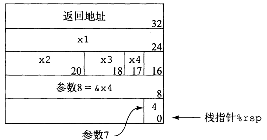
图 3-33 函数 call_proc 的栈帧。该栈帧包含局部变量和两个要传递给函数 proc 的参数
