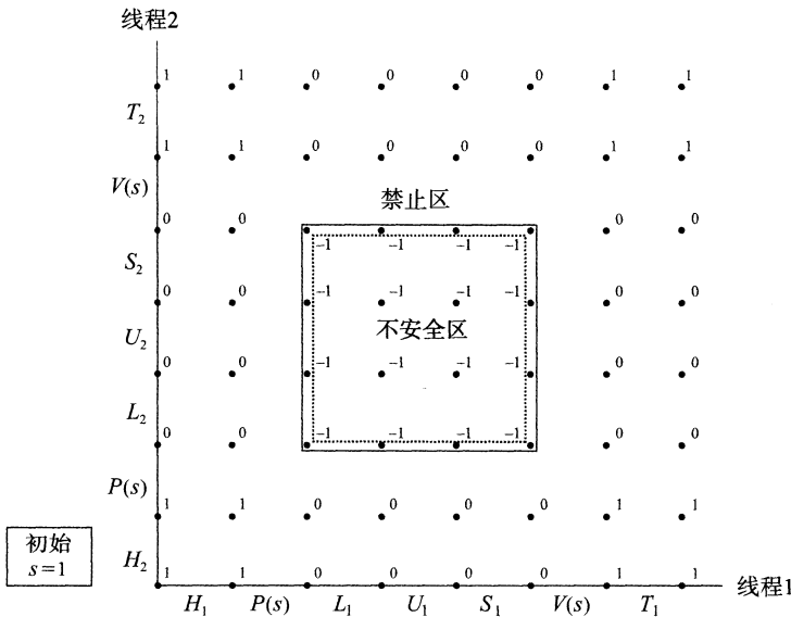
图 12-22 使用信号量来互斥。s < 0 的不可行状态定义了一个禁止区，禁止区完全包括了不安全区，阻止了实际可行的轨迹接触到不安全区
