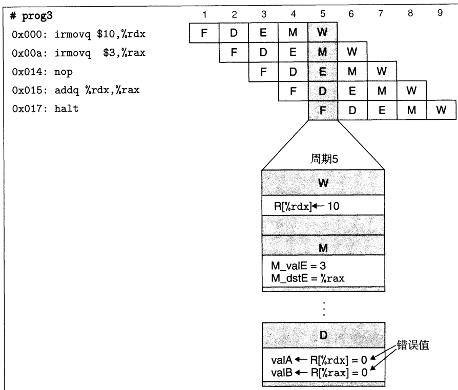
图 4-45 prog3 的流水线化的执行，没有特殊的流水线控制。在周期 5，addq 指令从寄存器文件中读源操作数。对寄存器 %rdx 的写仍处在写回阶段，而对寄存器 %rax 的写还在访存阶段。两个操作数 valA 和 valB 得到的都是错误值
