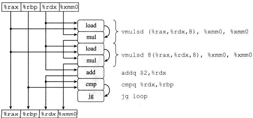
图 5-18 combine5 内循环代码的图形化表示。每次迭代有两条 vmulsd 指令，每条指令被翻译成一个 load 和一个 mul 操作
