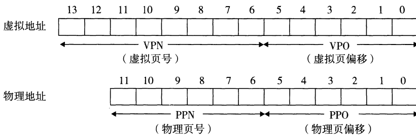
图 9-19 小内存系统的寻址。假设 14 位的虚拟地址( n=14 )，12 位的物理地址( m=12 )和 64 字节的页面( P=64 )
