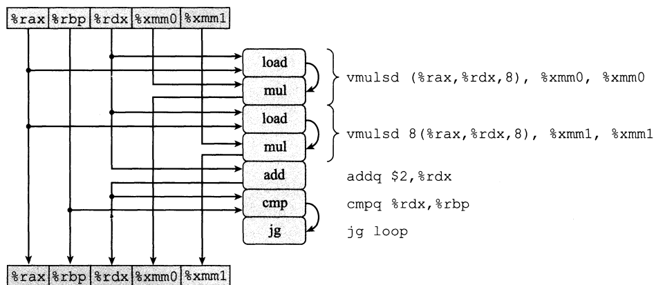
图 5-22 combine6 内循环代码的图形化表示。每次循环有两条 vmulsd 指令，每条指令被翻译成 load 和 mul 操作
