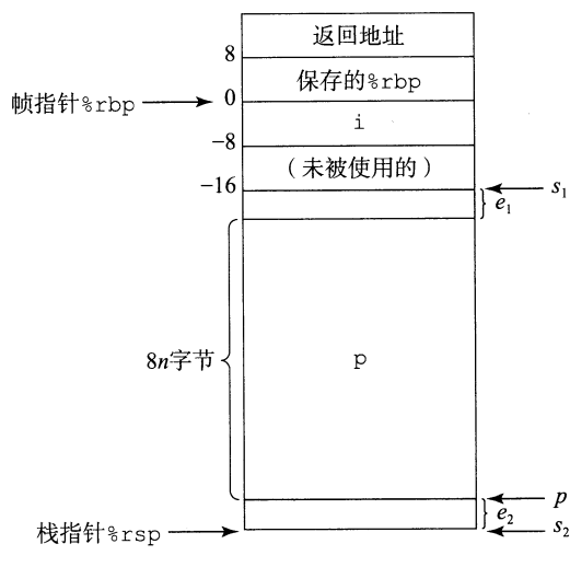
图 3-44 函数 vframe 的栈帧结构 (该函数使用寄存器 %rbp 作为帧指针。图右边的注释供练习题 3.49 所用)
