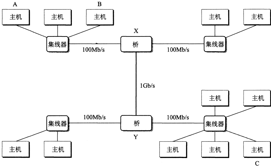
图 11-4 桥接以太网
