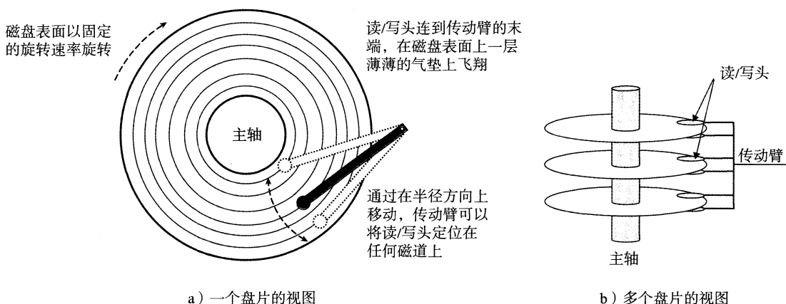
图 6-10 磁盘的动态特性
