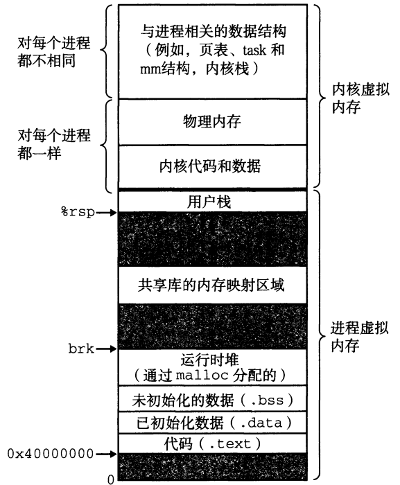
图 9-26 一个 Linux 进程的虚拟内存
