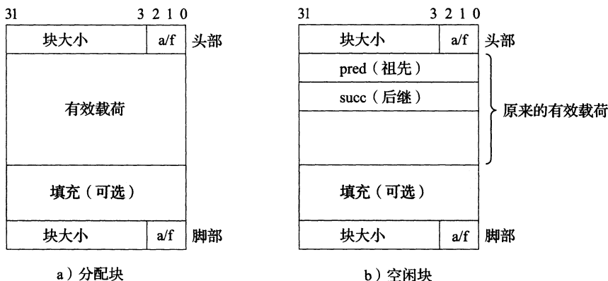
图 9-48 使用双向空闲链表的堆块的格式
