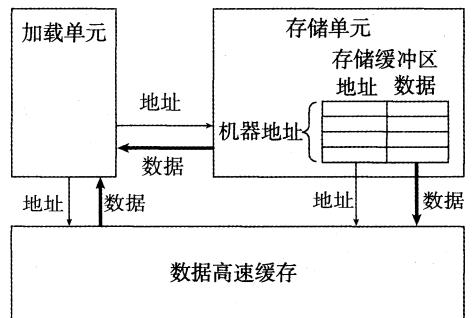
图 5-34 加载和存储单元的细节。存储单元包含一个未执行的写的缓冲区。加载单元必须检查它的地址是否与存储单元中的地址相符，以发现写/读相关
