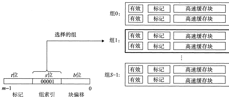
图 6-33 组相联高速缓存中的组选择
