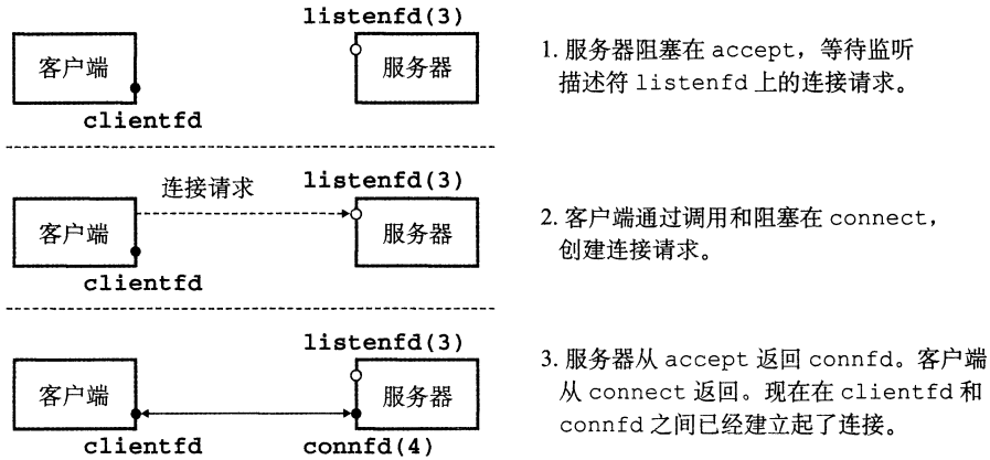
图 11-14 监听描述符和已连接描述符的角色
