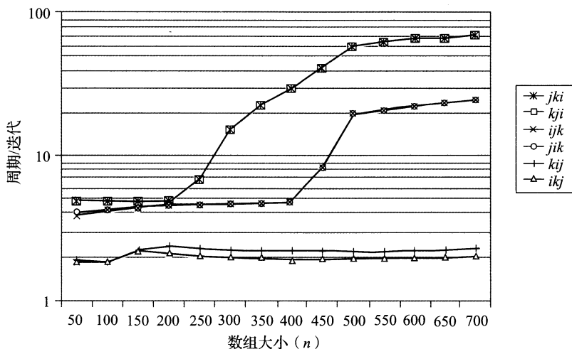
图 6-46 Core i7 矩阵乘法性能
