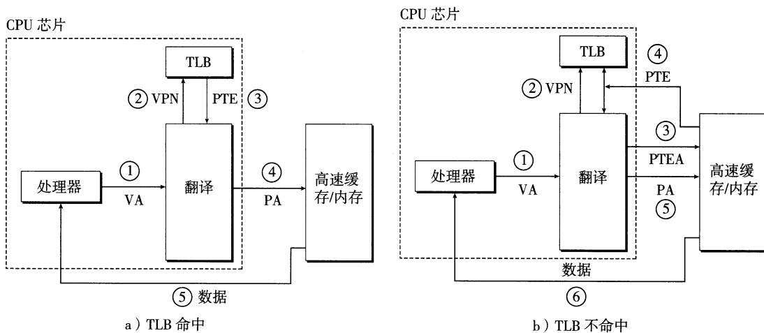
图 9-16 TLB 命中和不命中中的操作图
