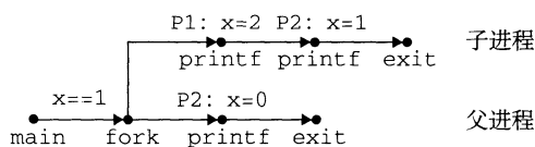
图 8-47 练习题 8.2 的进程图
