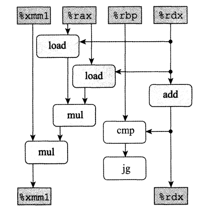
a) 重新排列、简化和抽象图5-27的表示，给出连续迭代之间的数据相关
