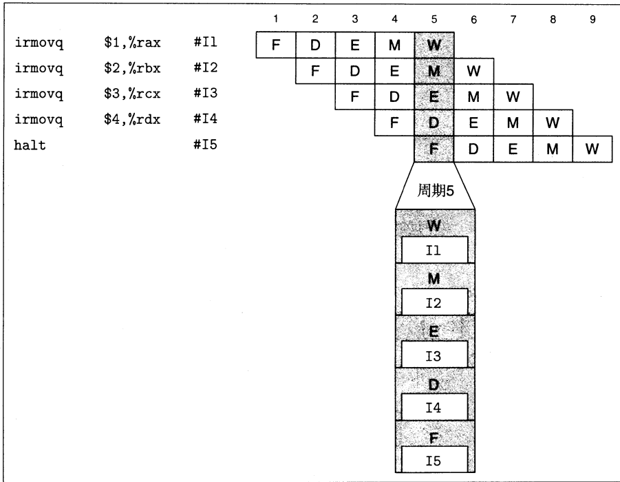
图 4-42 指令流通过流水线的示例
