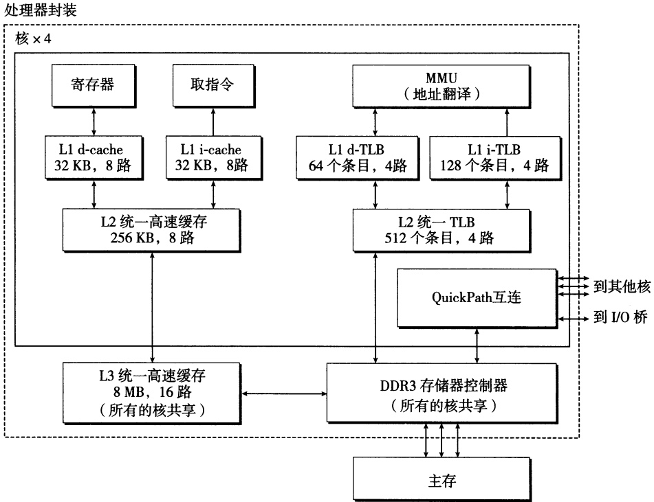
图 9-21 Core i7 的内存系统
