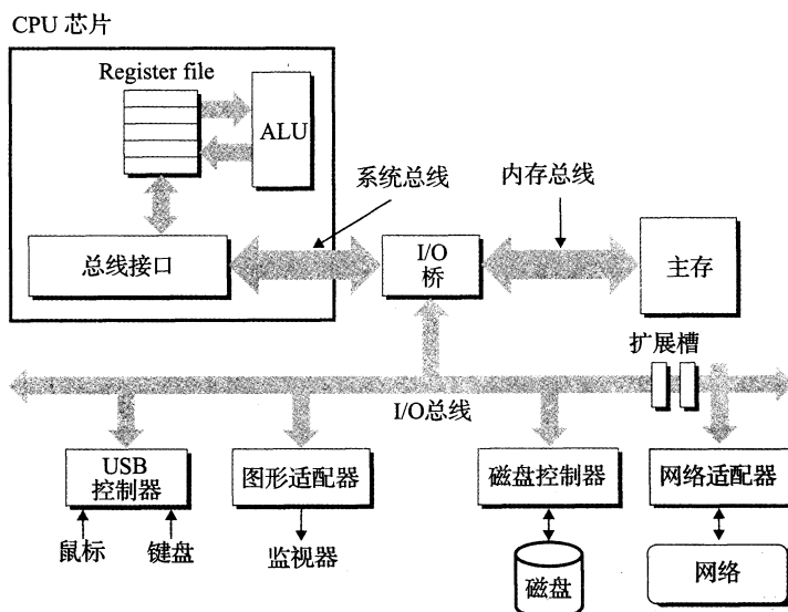
图 11-2 一个网络主机的硬件组成
