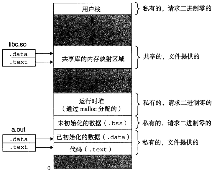
图 9-31 加载器是如何映射用户地址空间的区域的
