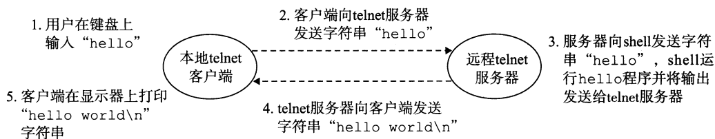
图 1-15 利用 telnet 通过网络远程运行 hello
