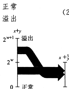
图 2-22 整数加法和无符号加法间的关系。当 x+y 大于 2^w - 1 时，其和溢出
