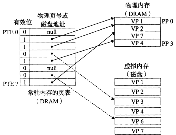
图 9-1 页表
