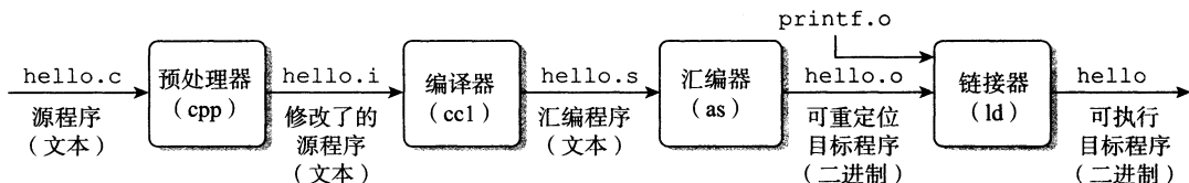
图 1-3 编译系统
