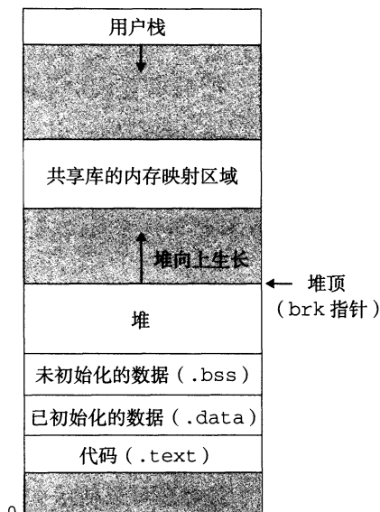
图 9-33 堆
