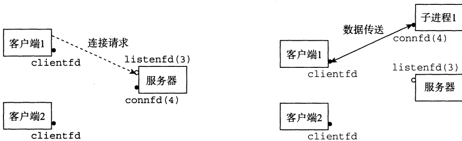
图 12-1 第一步：服务器接受客户端的连接请求 图 12-2 第二步：服务器派生一个子进程为这个客户端服务
