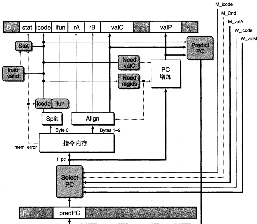
图 4-57 PIPE 的 PC 选择和取指逻辑。在一个周期的时间限制内，处理器只能预测下一条指令的地址
